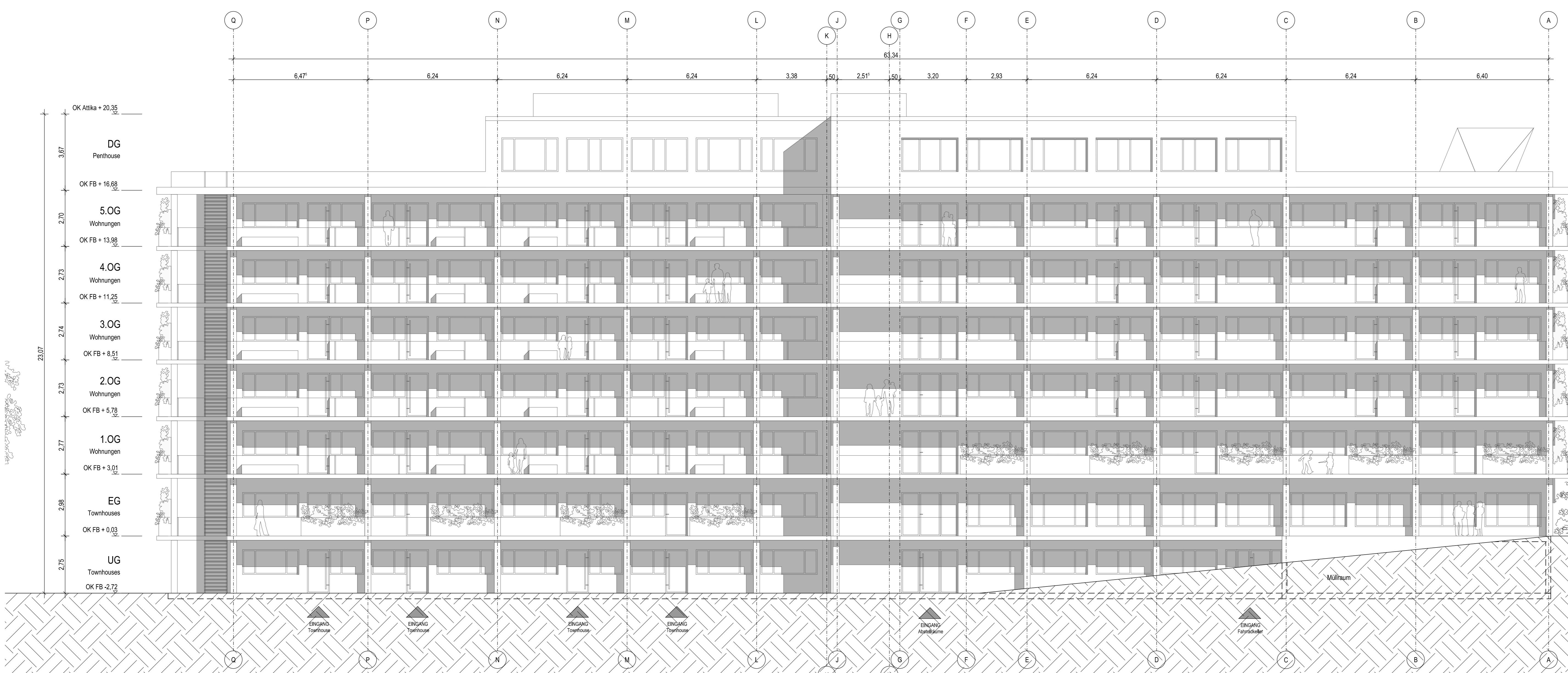
ANSICHT NORD-OST (SALINE)
