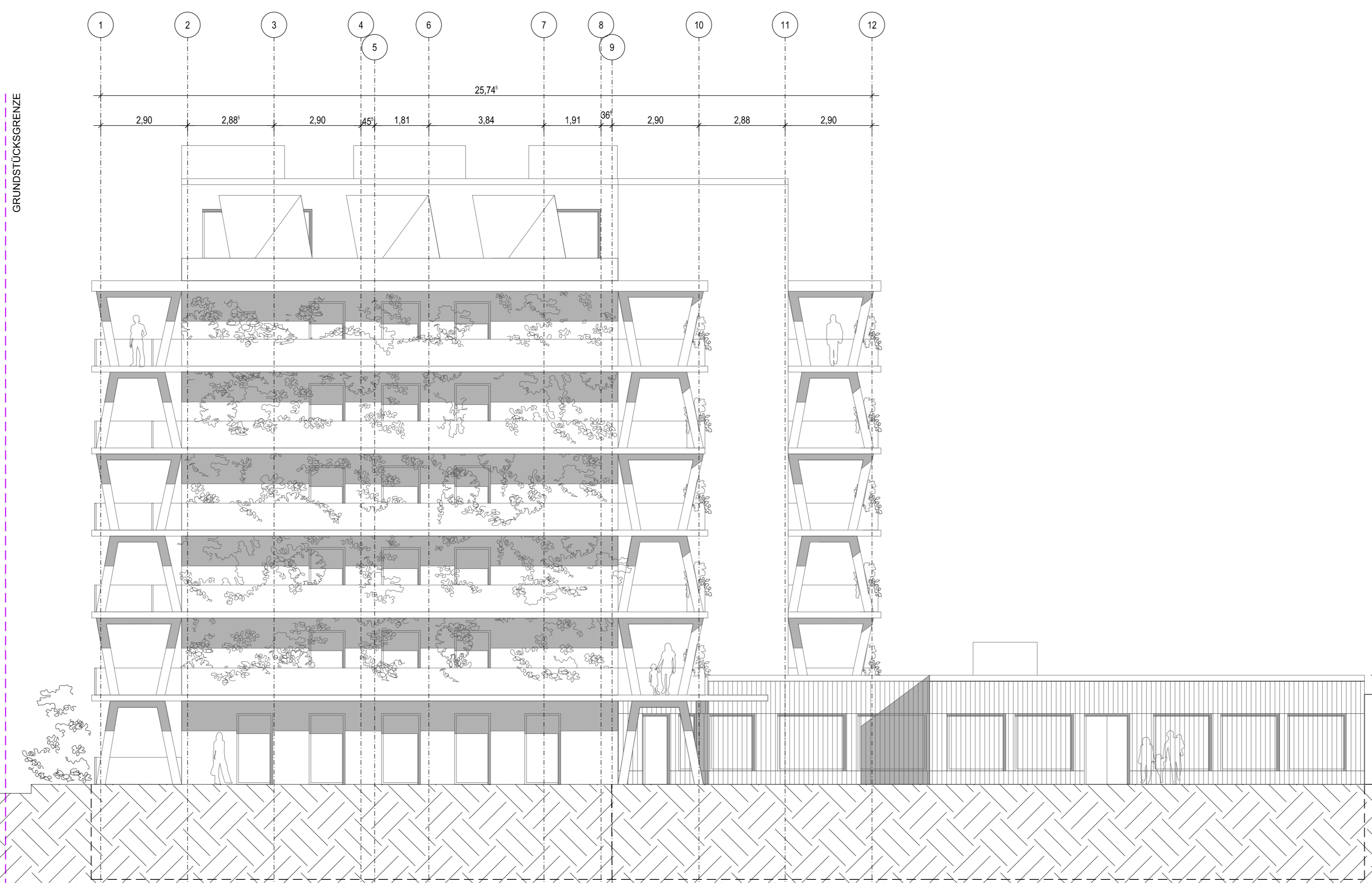
ANSICHT NORD-WEST (KURHAUSSTRASSE)
