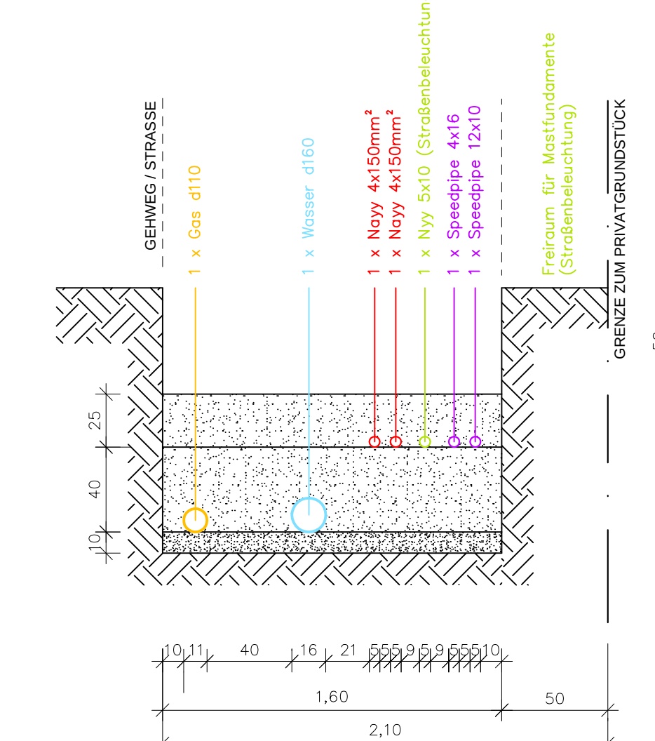
Grabenquerschnitt alle Versorgungsleitungen M 1:25
