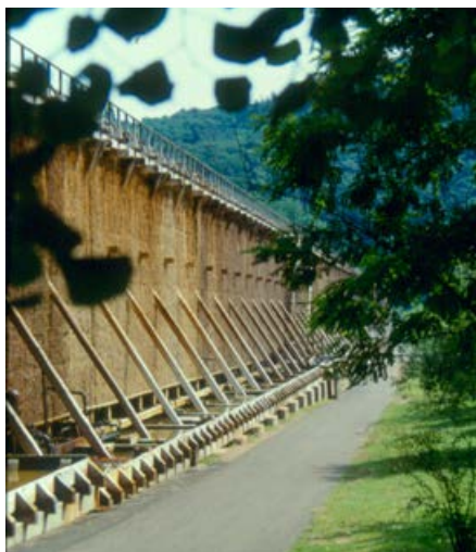
Gradierwerke
