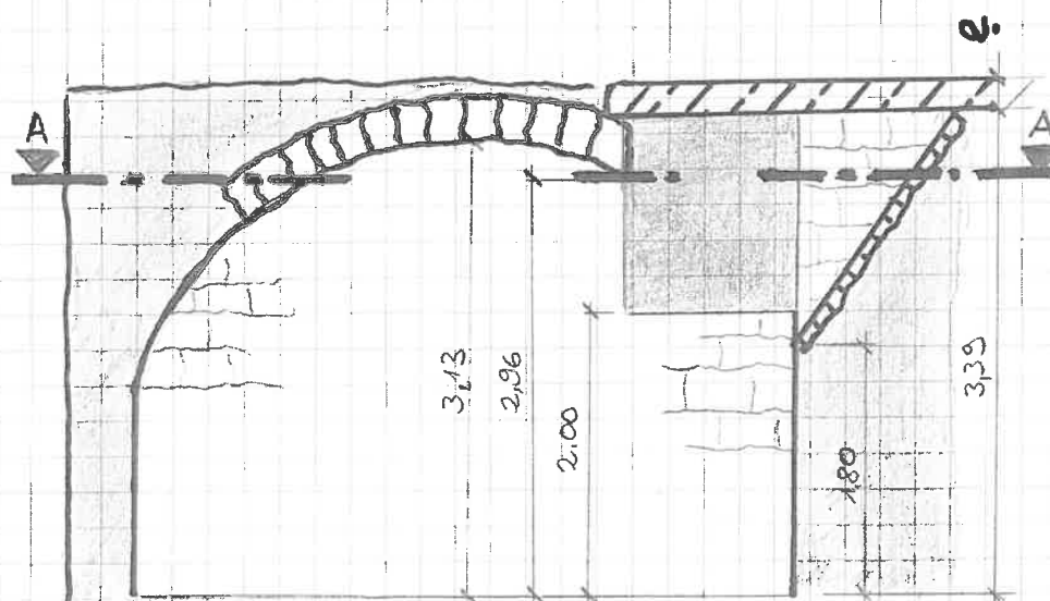
Schnitt B-B
